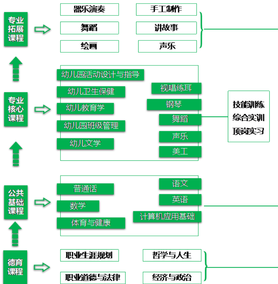
图 1 课程结构图
